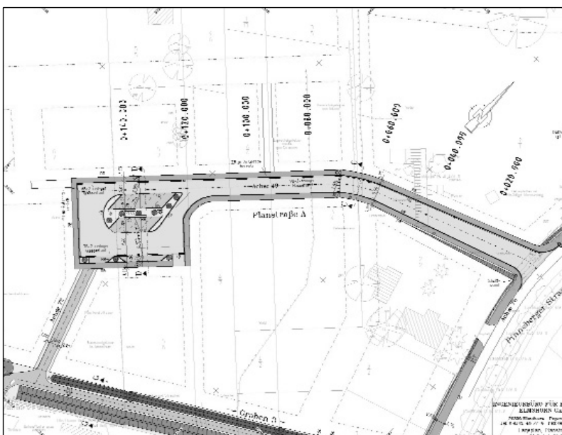
Lageplan Stichstraße A (Asphaltbauweise)
