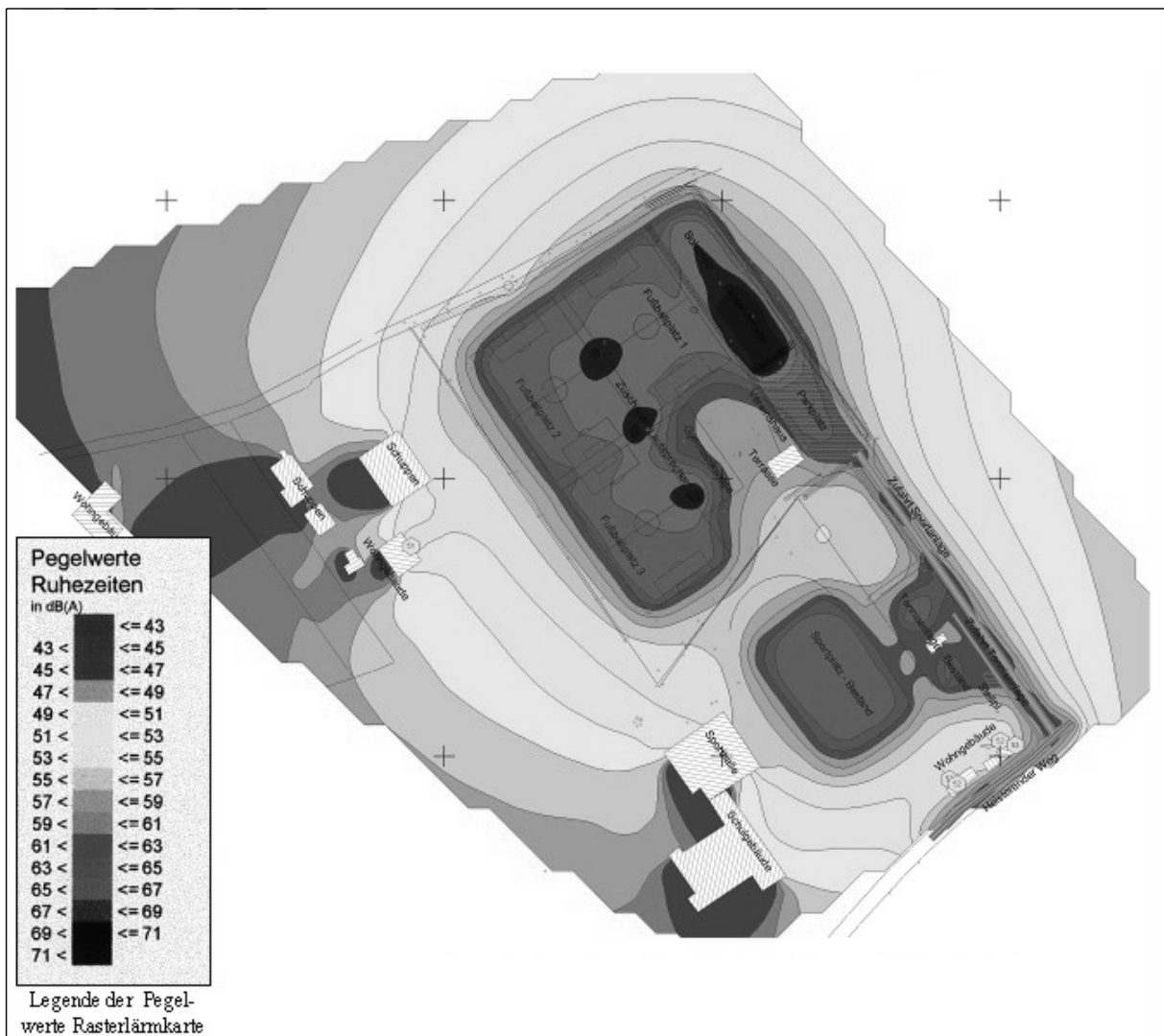
Rasterlärmkarte Sportanlage: Maximaler Belastungsfall ohne Erdwall
