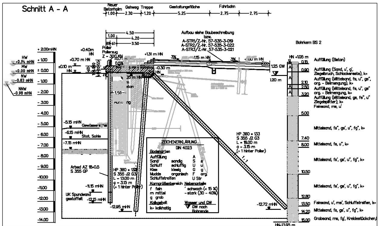
Schnitt durch die Spundwand und Rückverankerung
